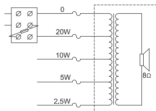
Diagrama do circuito
