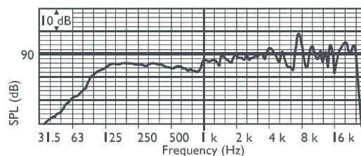
Frequência de resposta
